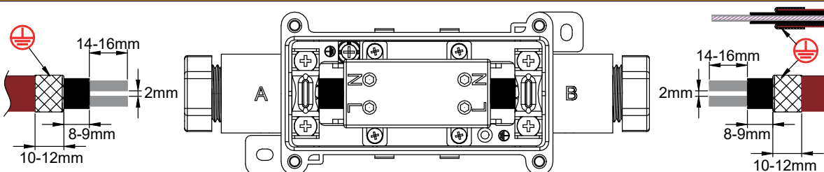
Modèle à deux câbles chauffants (Y502)
