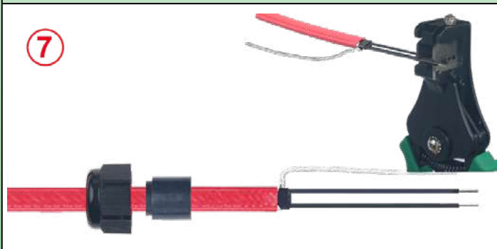
7 : Dénuder la partie semi-conductrice restante à l'extrémité des deux conducteurs, sur la longueur requise.
