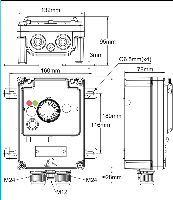
Modèle à 3 presse-étoupes (2 × M24 + 1 × M12) : Y8WR-X
