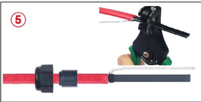
5 : Dégainer la couche isolante électrique sur la longueur requise.
