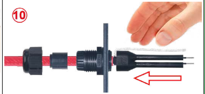
10 : Glisser les manchons isolants sur les conducteurs des câbles chauffants, en laissant le conducteur de terre en dehors, ou avec le conducteur à l'intérieur, si le manchon est à trois conducteurs
