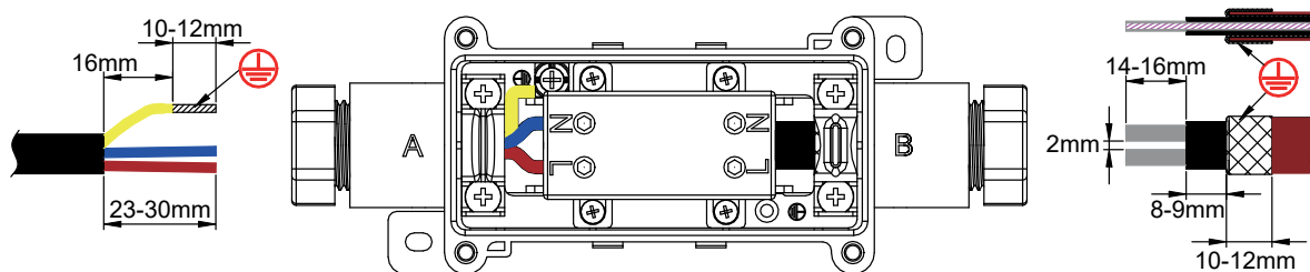
Modèle à un câble chauffant et un câble d'alimentation (Y501)
