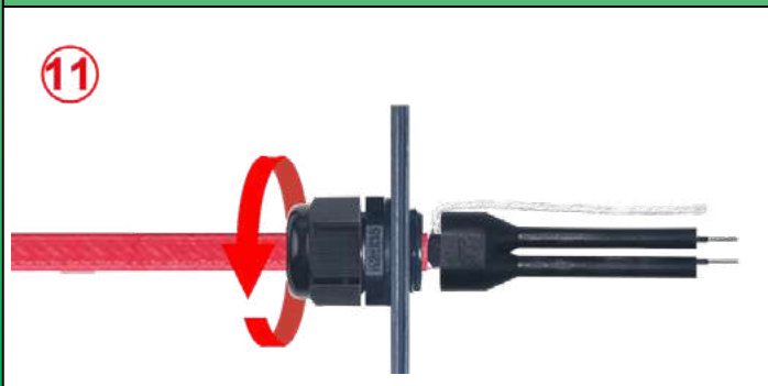
11 : Serrer l'écrou du presse étoupe sur le joint d'étanchéité
