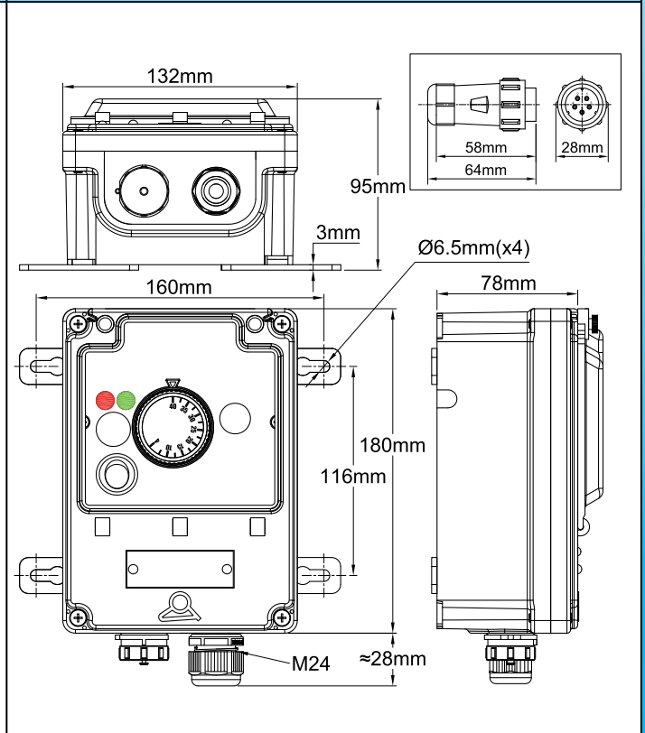
Modèle à un connecteur 5 voies et un presse-étoupe M24 : Y8WR-Y
