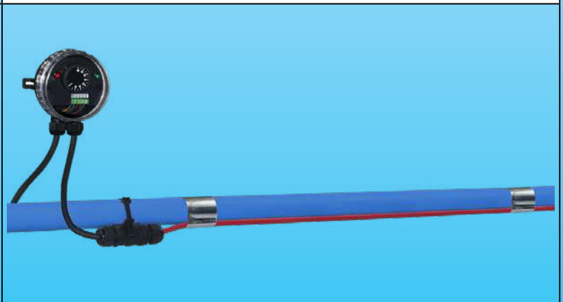
Exemple de montage en commande d'un câble chauffant pour mise hors gel d'un tuyau en PVC, combiné avec un boîtier Y24.
