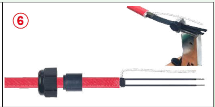
6 : Couper la partie chauffante entre les deux conducteurs sur la longueur requise.
