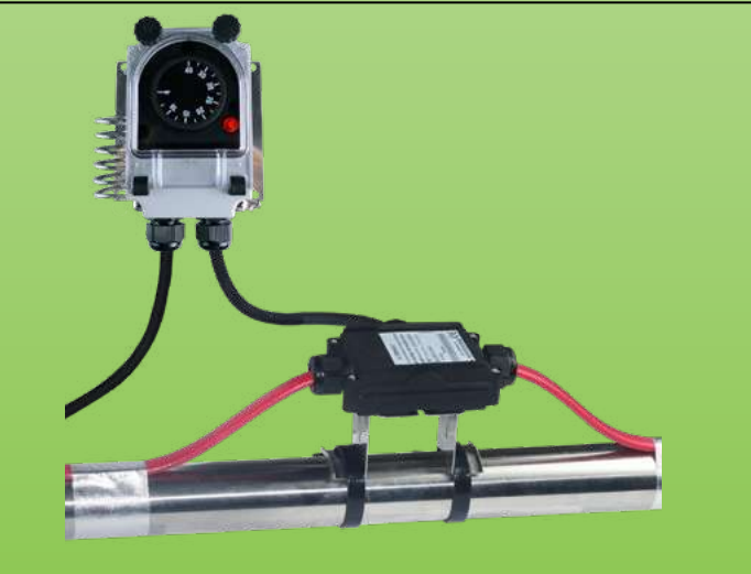
Exemple de montage en commande de deux câbles chauffants pour mise hors gel d'un tuyau en acier, combiné avec un boîtier Y27.
